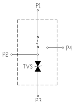
热保护型瞬态抑制二极管 (机械脱扣型)
