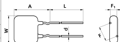
直型引线 Straight Lead
