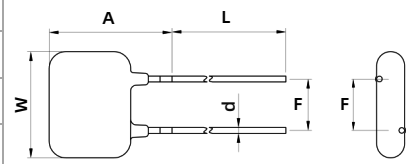
外弯型引线 Outward Crimp
