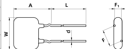
内弯型引线 Inward Crimp
